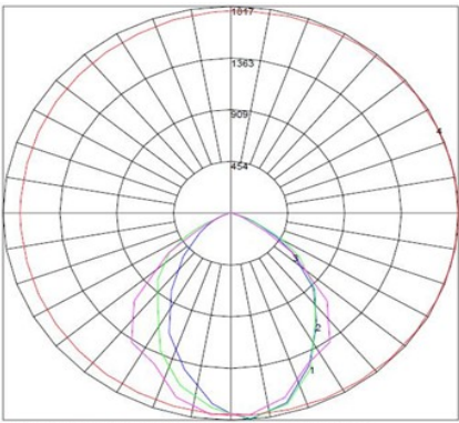
MHT-GRW-55E
