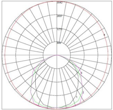
MHT-GRW-150E
