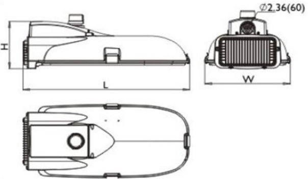
MHT-GRW-40-250E
